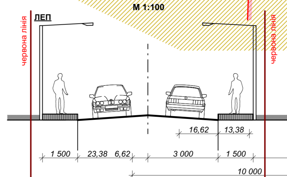
Поперечний профіль вул. Нова, вул. П. Українки, вул. Галицька, вул. Проєктована №1, вул. Проєктована №2, М 1:100
